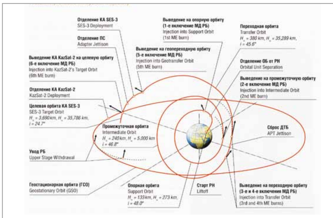
Схема полета РН «Протон-М», РБ «Бриз-М» при выведении SES-3 и KazSat-2 на целевые орбиты Proton-M / Breeze-M System Trajectory
